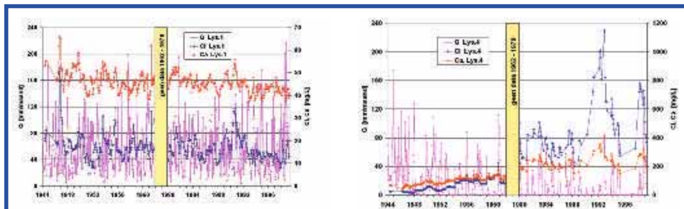
Afb. 3: Verloop van de afvoer en concentratie calcium en chloride in drainagewater van lysimeter 1 (onbegroeid) en 4 (dennen) te Castricum.
