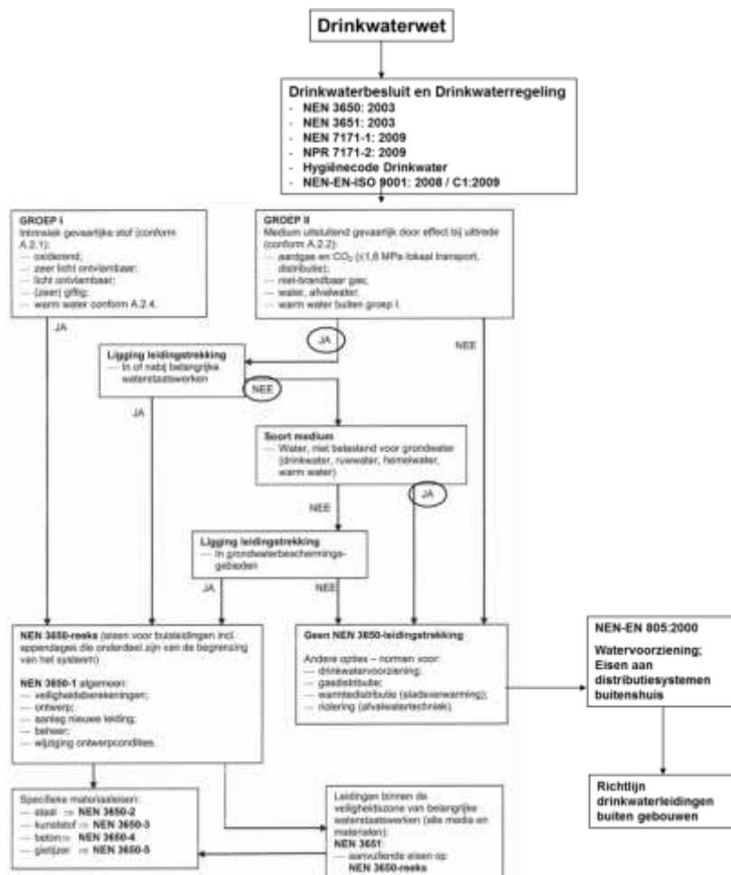
Figuur 1 'Stroomschema groepsindeling en normen' uit NEN 3650-1 , uitgebreid met de Drinkwaterwet, het Drinkwaterbesluit, de Drinkwaterregeling, de NEN-EN 805 en de onderhavige richtlijn.
