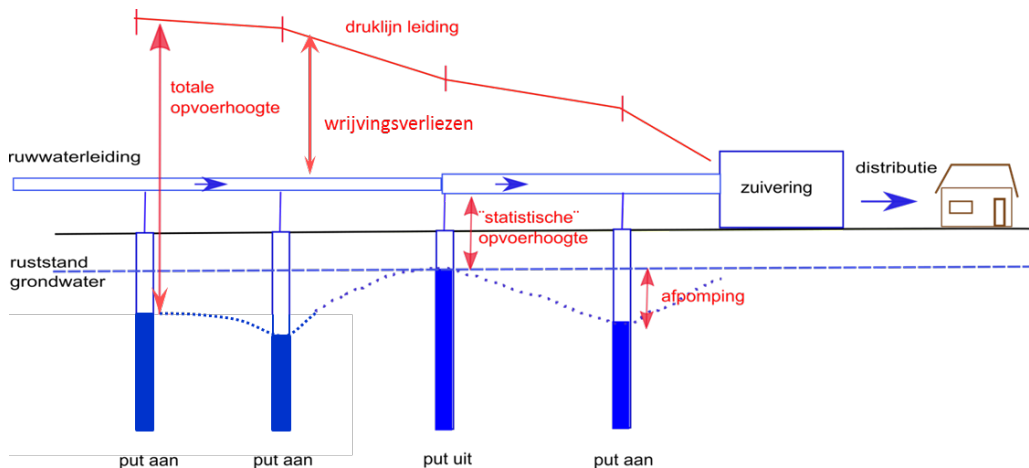
Figuur 2-1 De totale opvoerhoogte van een winveld is opgebouwd uit wrijvingsverlies in de leiding, de "statische" opvoerhoogte en de afpompingsverlies van putten.
