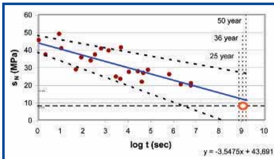
Afb. 8: Gemeten weerstand tegen langzame scheurgroei.
