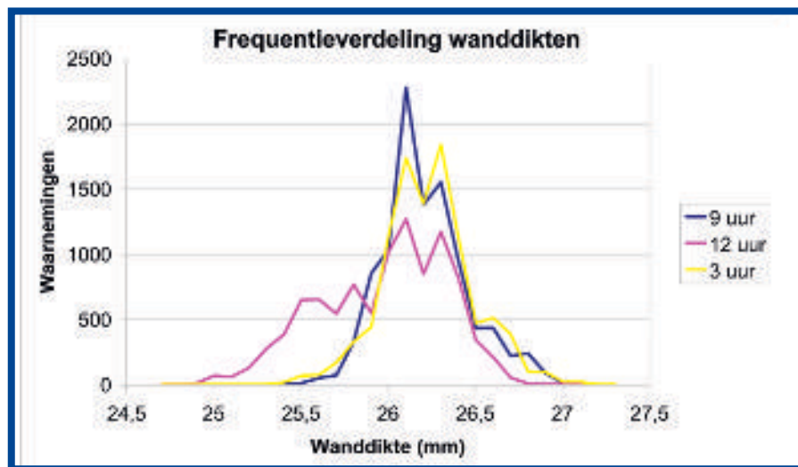
Afb. 3: Resultaten georadar op verschillende klokstanden.
