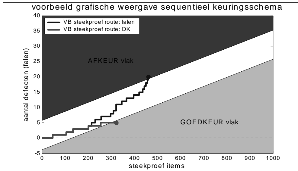
Figuur II-1 voorbeeld sequentieel keuringsschema
