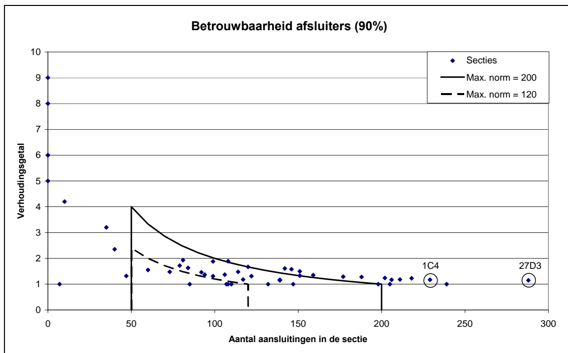
figuur 5 De verhoudingsgetallen van de door een breuk getroffen secties uitgezet tegen het oorspronkelijk aantal aansluitingen (bij een afsluiterbetrouwbaarheid van 90%)
