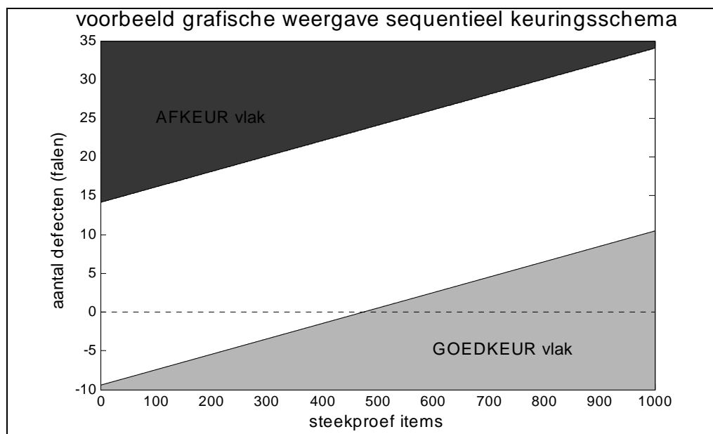
Figuur II-2 Sequentieel keuringsschema bij \beta = 0,025
