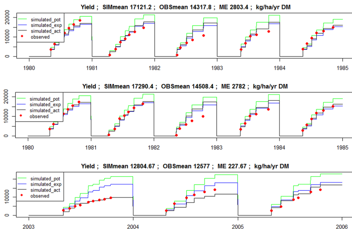
FIGUUR 4.2 MODELRESULTATEN EN METINGEN VAN GEWASOPBRENGSTEN VOOR GRASLAND: BOVEN RUURLO16 (A), MIDDEN RUURLO48 (B), EN ONDER ZEGVELD03 (C). GROEN: BEREKENDE POTENTIËLE OPBRENGST, BLAUW: DE BEREKENDE EXPLOITEERBARE OPBRENGST, ZWART: DE BEREKENDE ACTUELE OPBRENGST, ROOD: DE GEMETEN OPBRENGST.
