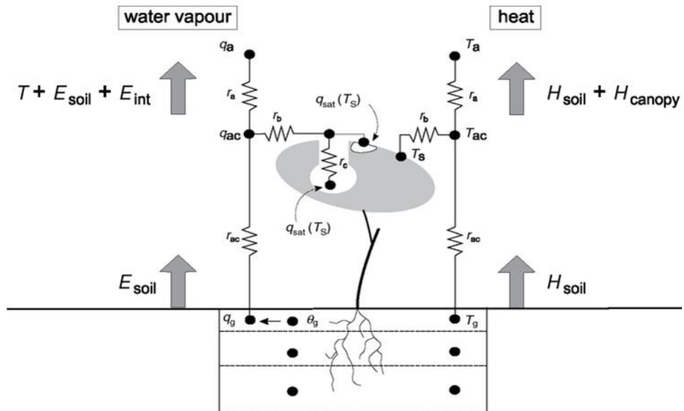
FIGUUR 2.5 SVAT SCHEMA MET WEERSTANDEN VOOR WATER- EN WARMTE-TRANSPORT (MOENE EN VAN DAM, 2014)
