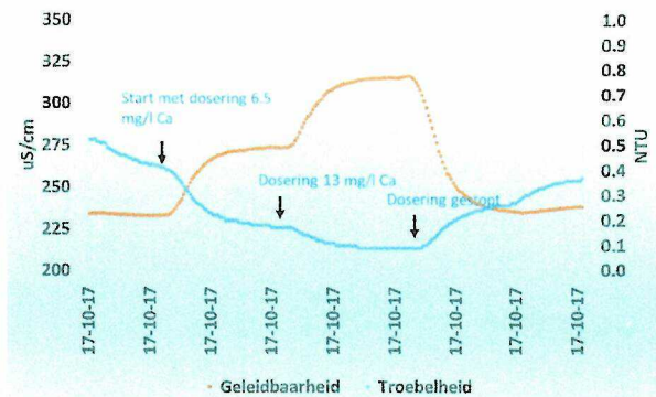
Afbeelding 3: Troebelheid en geleidbaarheid filtraat in relatie tot gedoseerd Ca aan ruw 2
