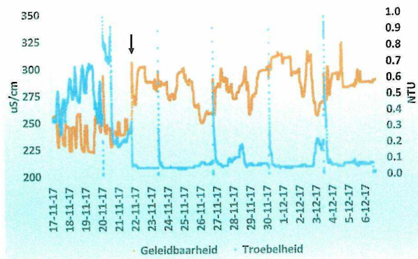
Afbeelding 1: Troebelheid filtraat in relatie tot geleidbaarheid ruw 1 en 2. De pijl geeft het punt aan van overschakelen van ruw 2 naar ruw 1
