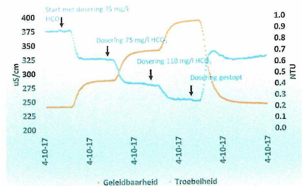
Afbeelding 2: Troebelheid en geleidbaarheid filtraat in relatie tot gedoseerd \text{HCO}_3^- aan ruw 2
