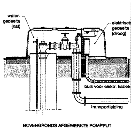
Figuur 8-5 Bovengronds afgewerkte pompput. (SBW, 1995)
