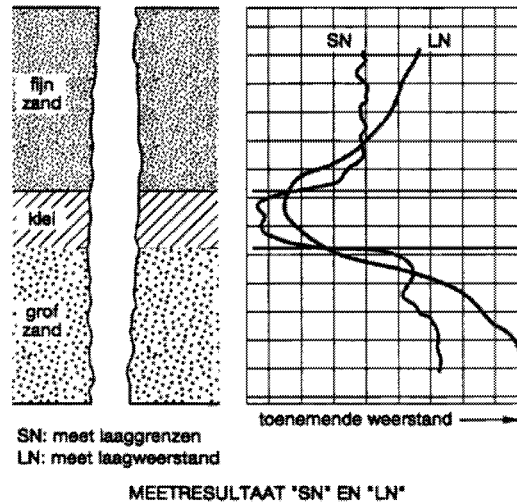
Figuur 11-6 Meetresultaat 'SN' en 'LN'. (SBW, 1997)
