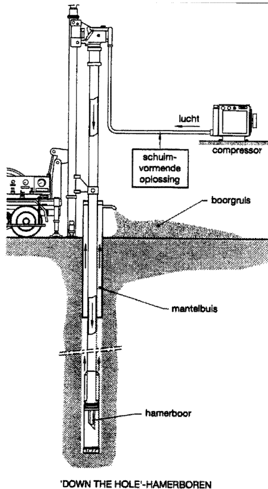
Figuur 6-9 'Down the hole'-hamerboren. (SBW, 1995)
