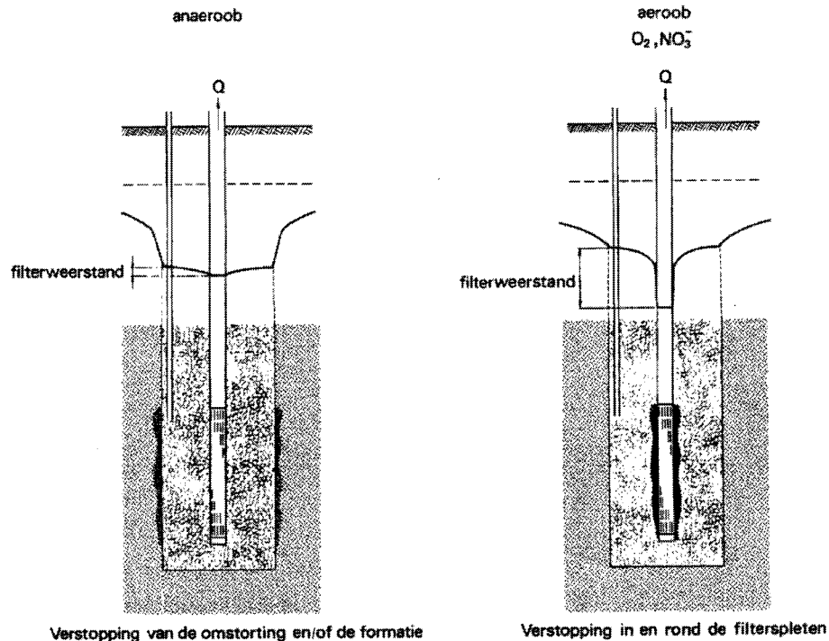
Figuur 15-4 De twee vormen van putverstopping (SBW, 1997).
