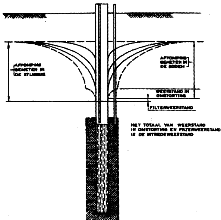
Figuur 15-2 Afpompingswaarde en intreeweerstand (SBW, 1995).
