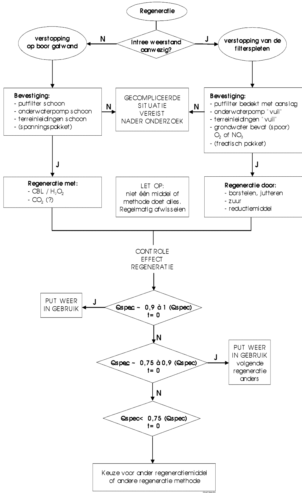
Figuur 15-6 Stroomschema uitvoering regeneratie.
