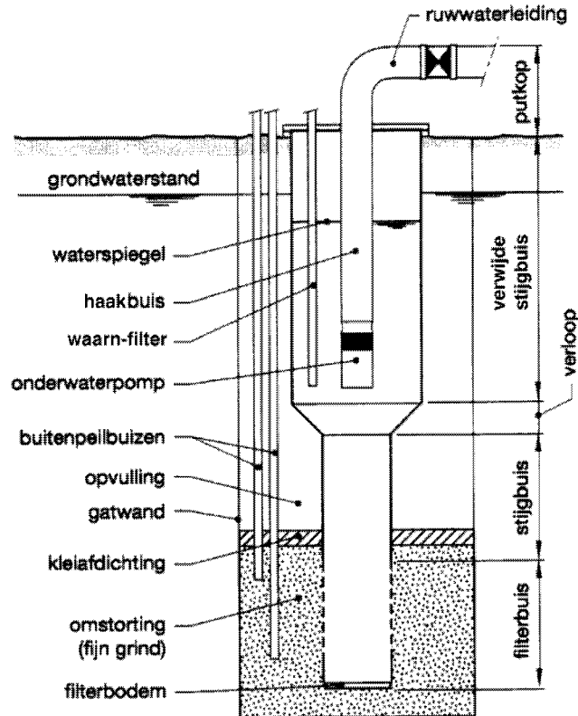
OPBOUW POMPPUT
