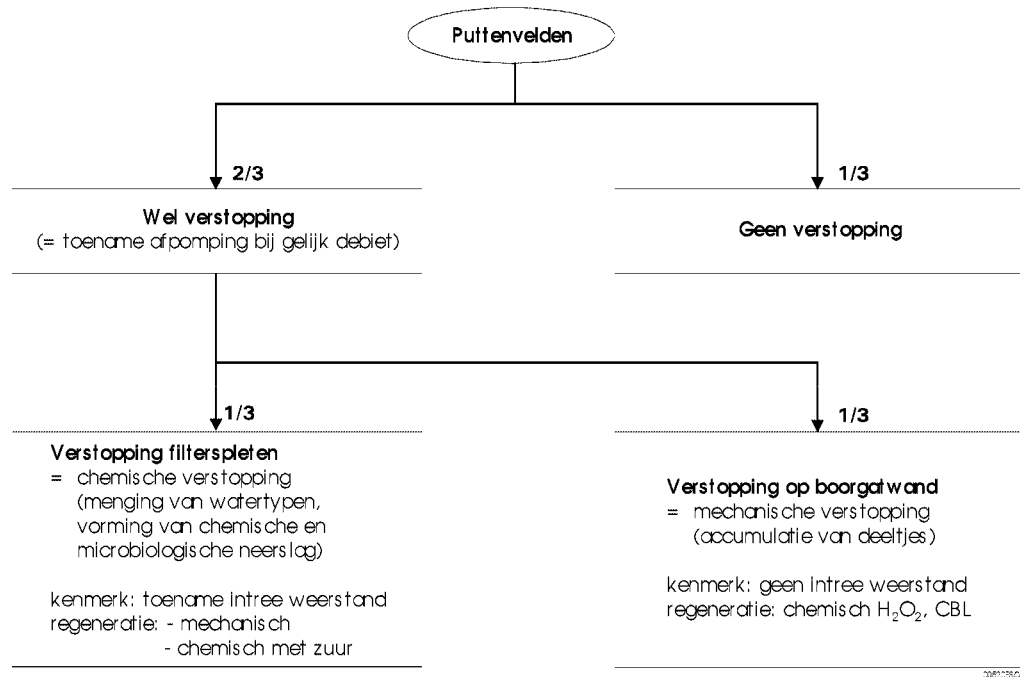
Figuur 15-1 Stroomschema voor het vaststellen van putverstopping en methoden voor regeneratie
