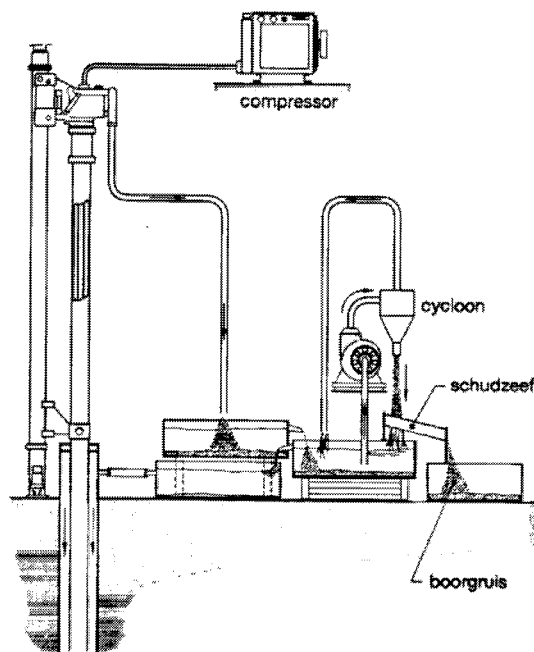
LUCHTLIFTEN MET CYCLOON EN SCHUDZEEF
