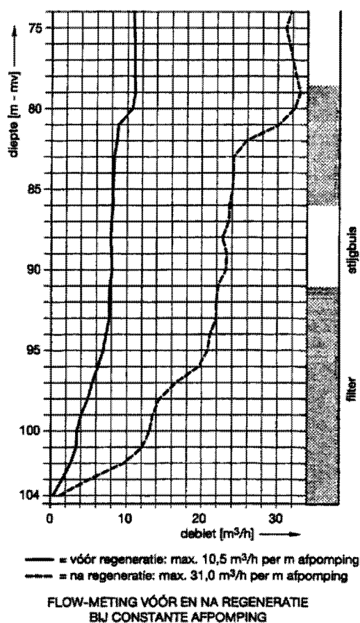
Figuur 11-8 Flow-meting vóór en na regeneratie bij constante afpomping. (SBW, 1997)
