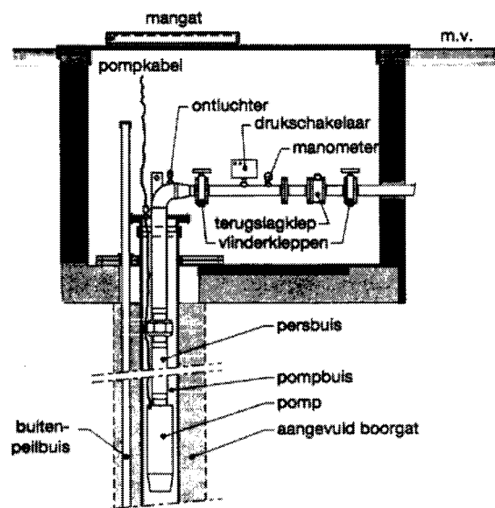
BETONNEN PUTKELDER MET POMP
