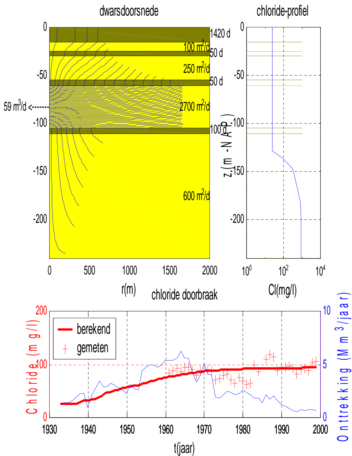
Figuur 7-4 Resultaat van een berekening waarmee een eerste inschatting van het risico van verzilting wordt bepaald.
