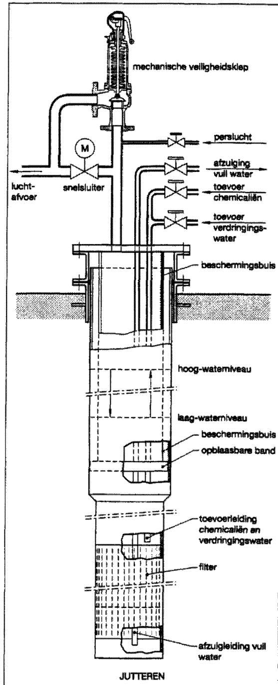
Figuur 15-7 Jutteren (SBW, 1997).
