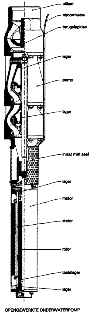
Figuur 8-3 Onderwaterpomp. (SBW, 1997)
