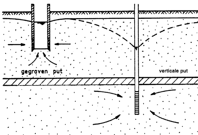
Grondwateronttrekking met verticale winmiddelen
