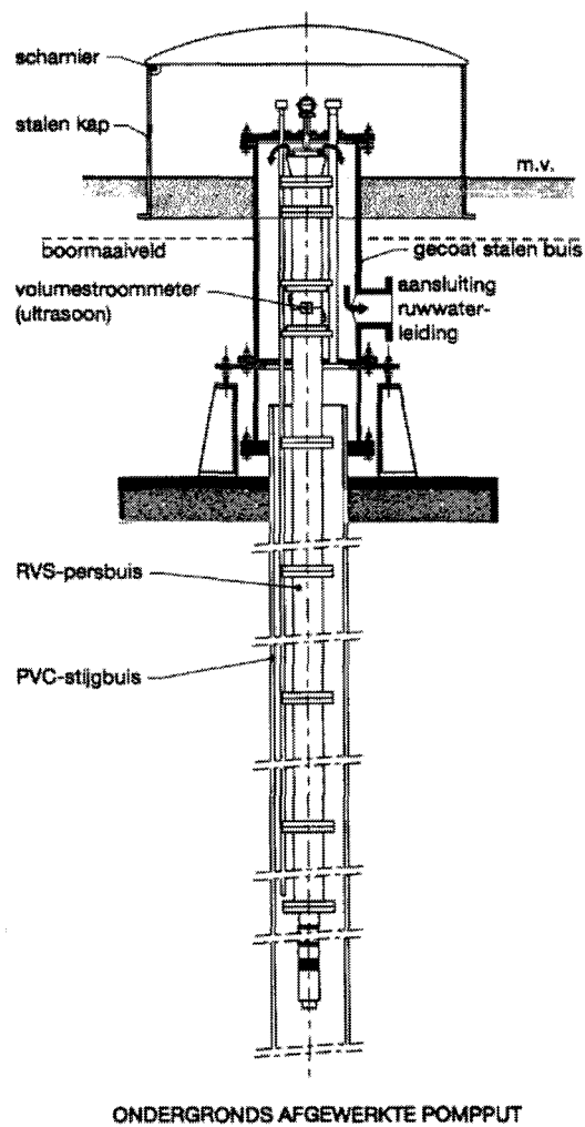
Figuur 8-4 Ondergronds afgewerkte pompput. (SBW, 1995)
