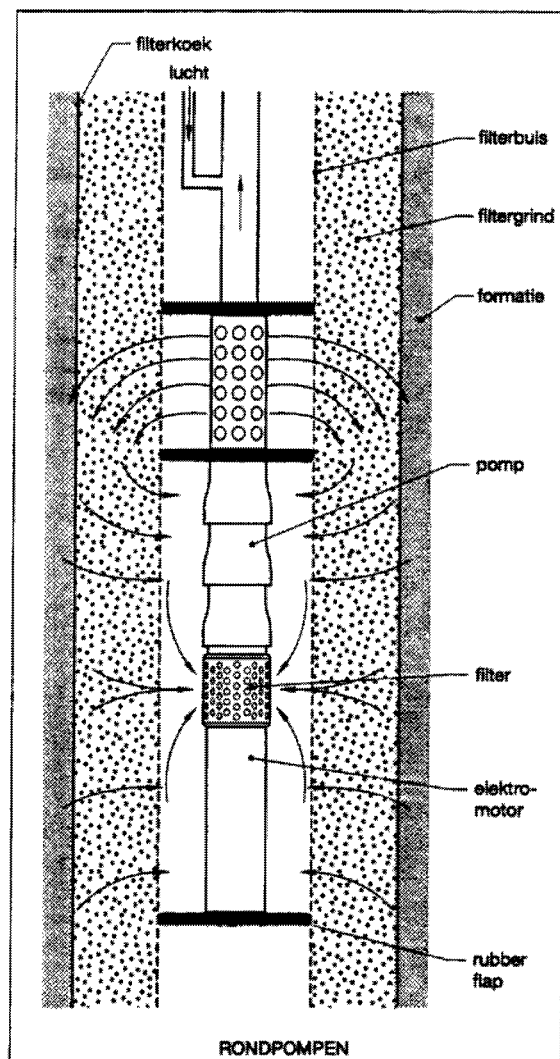
Figuur 15-8 Het principe van rondpompen. (SBW, 1997)
