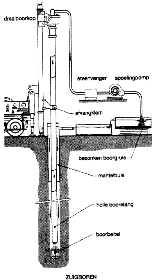
Figuur 6-6 Roterend zuigboren. (SBW, 1995)
