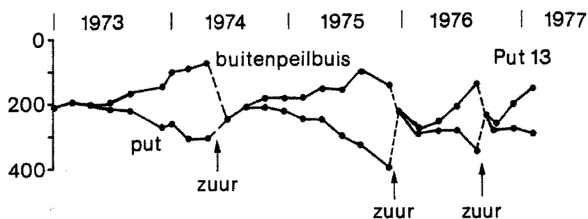
Figuur 15-3 Verloop stijghoogte in pompput en in buitenwaarnemingsbuis.
