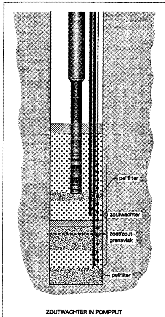
Figuur 16-1 Zoutwachter geplaatst in en pompput (SBW, 1997)
