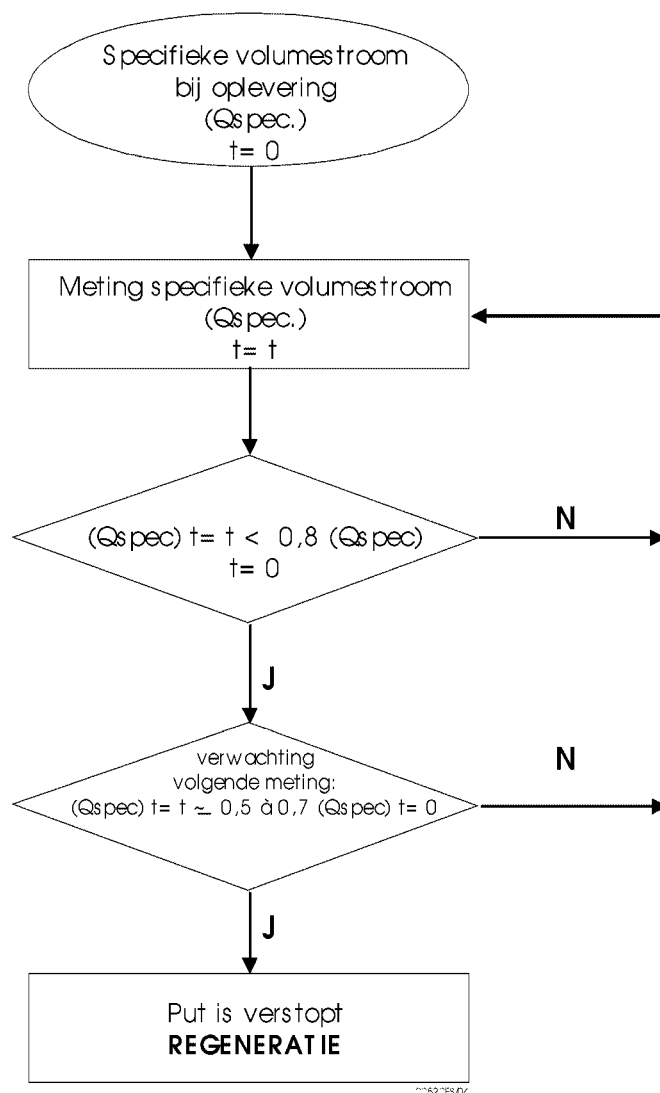
Figuur 15-5 Stroomschema voor vaststellen van putverstopping.
