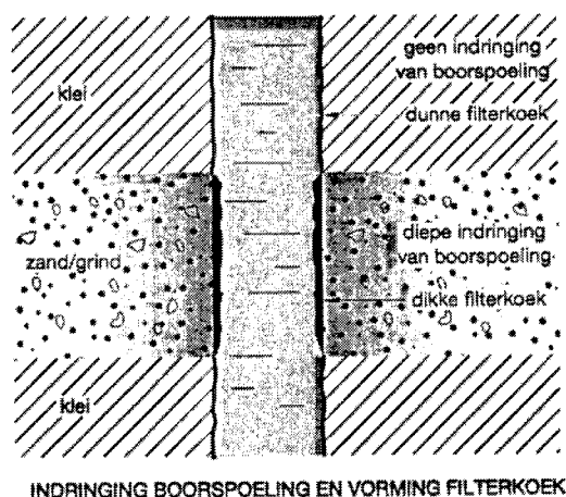
Figuur 11-1 Indringing boorspoeling en vorming filterkoek. (SBW, 1995)
