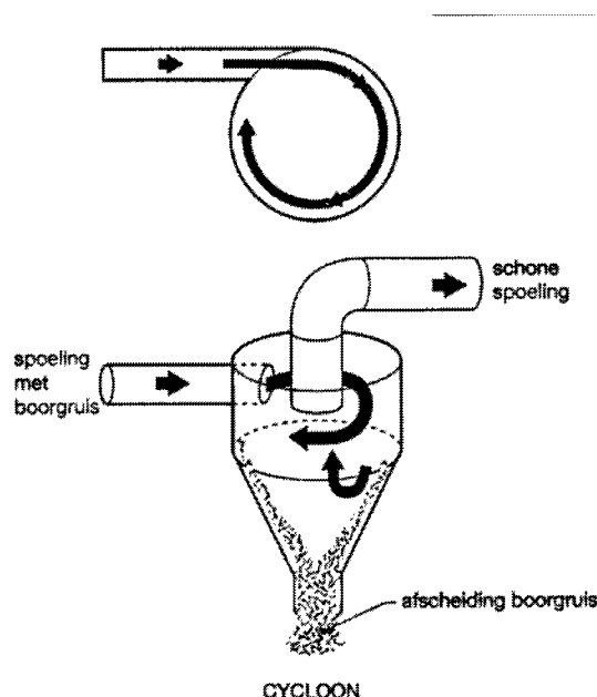
Figuur 11-2 Cycloon. (SBW, 1995)
