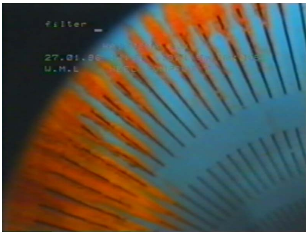
Foto 15-1 Verstopping van de filterspleten door ijzerneerslag (M. Juhász, WML )
