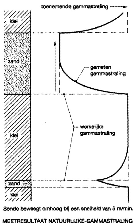
Figuur 11-7 Meetresultaat natuurlijke-gammastraling. (SBW, 1995)
