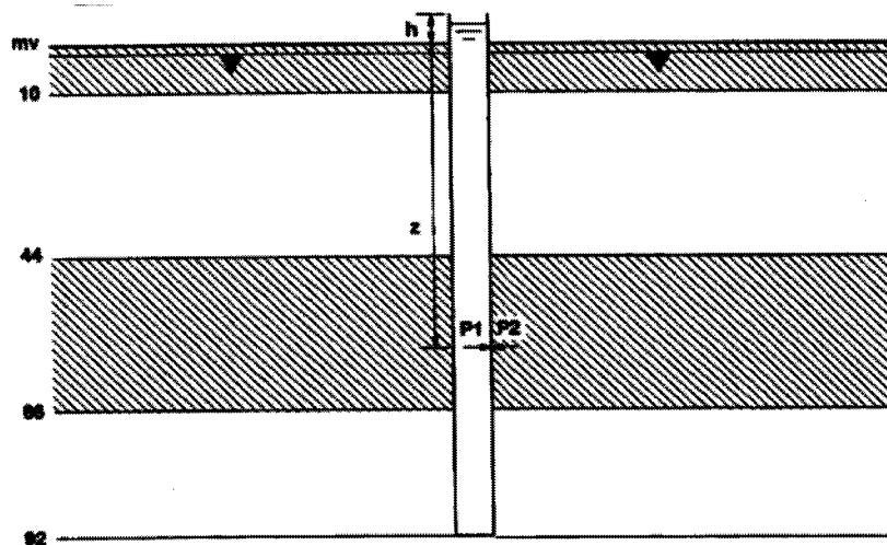
Figuur 7-2 Stabiel boorgat doordat P_1 \geq P_2
