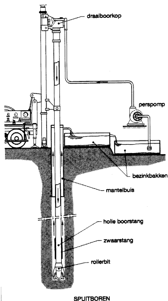
Figuur 6-7 Roterend spuitboren. (SBW, 1995)
