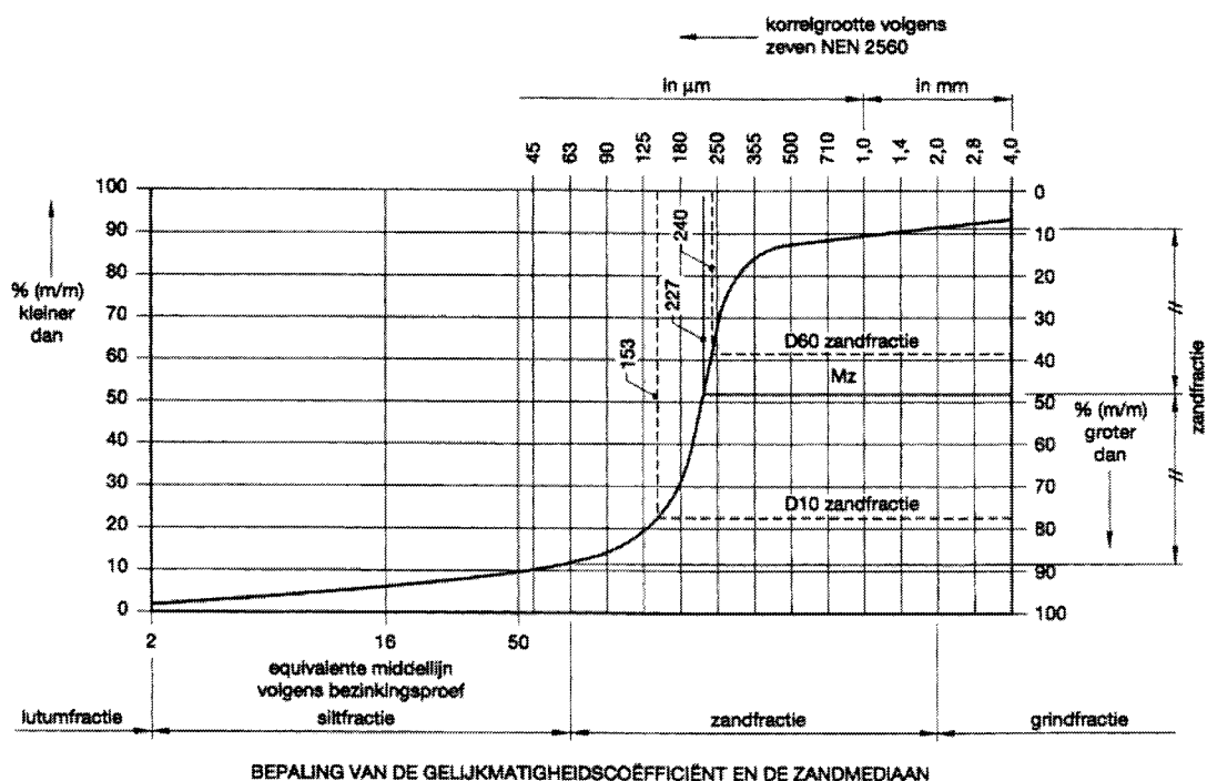
Figuur 8-2 Zeefkromme.
