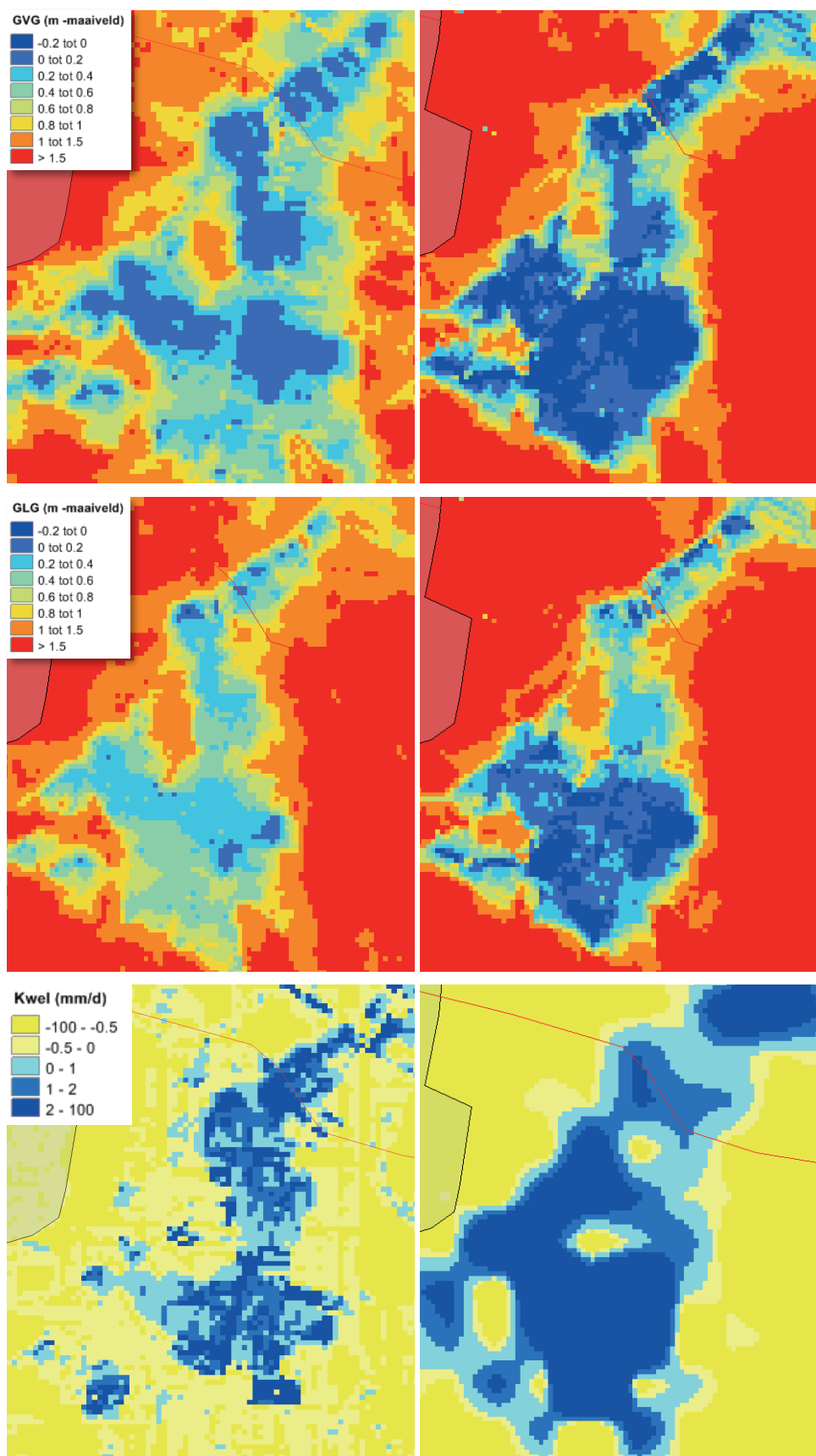
FIGUUR 54 VERGELIJKING UITKOMSTEN VAN HET BRABANT MODEL (LINKS) MET DE NEERGESCHAALDE UITKOMSTEN VAN HET NATIONALE HYDROLOGISCHE MODEL (RECHTS)
