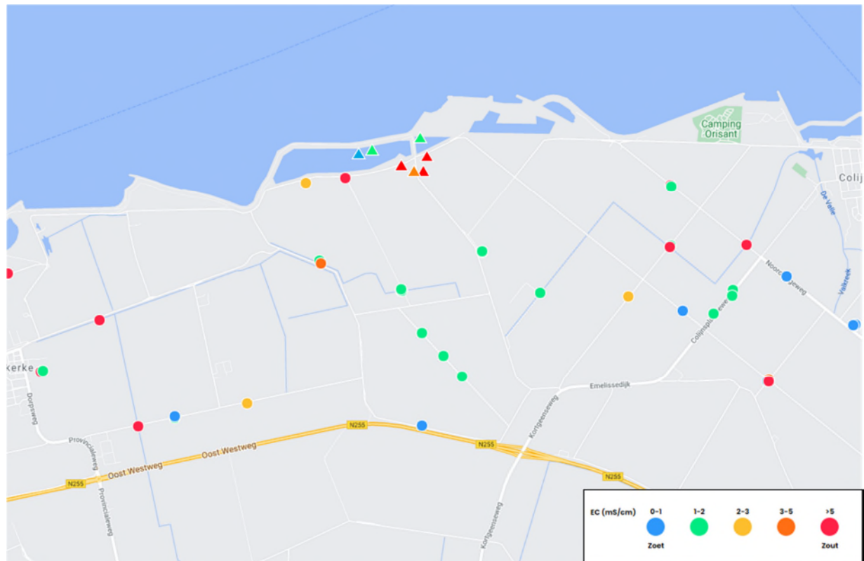
Figuur 4 EGV-metingen van het oppervlaktewater. Bollen: meetnet Noord-Beveland, situatie eind mei 2021; driehoeken: eigen metingen tijdens veldbezoek 27 mei 2021 (bron: dashboard Noordbevelandmeet.nl).
