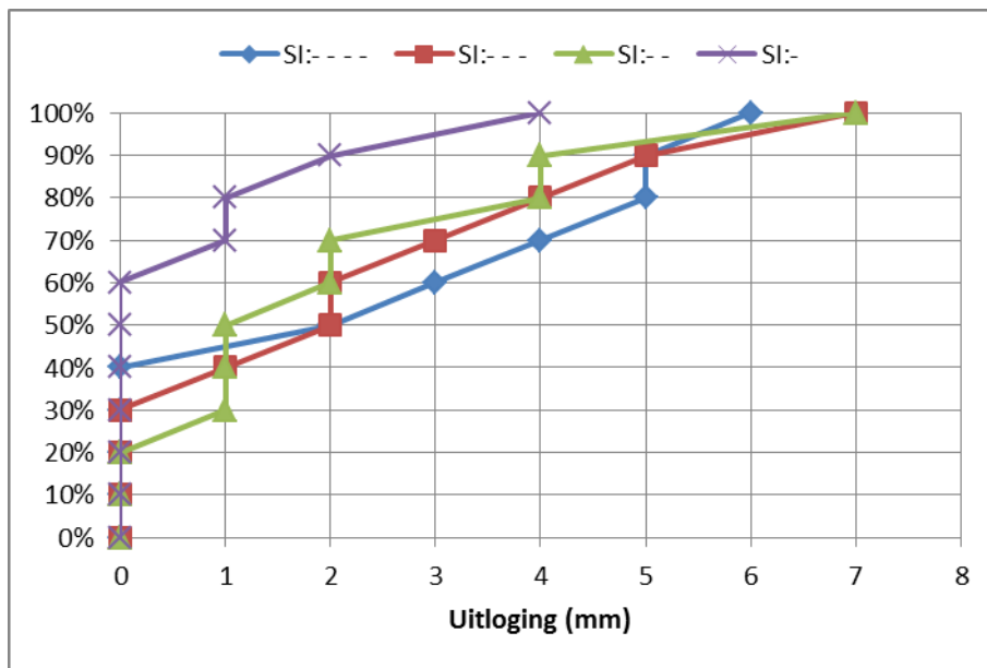
Figuur 6-12 Cumulatieve frequentieverdeling voor inwendige uitlogging in relatie tot het totaal aantal negatieve SI-dagen. De subgroepen zijn verkregen door de beoordelingen te sorteren en te verdelen in vier groepen van gelijke omvang. 'SI: - - - -' staat voor de 25% met de meest negatieve SI-waarde en 'SI: -' voor de 25% minst negatieve SI-waarden.
