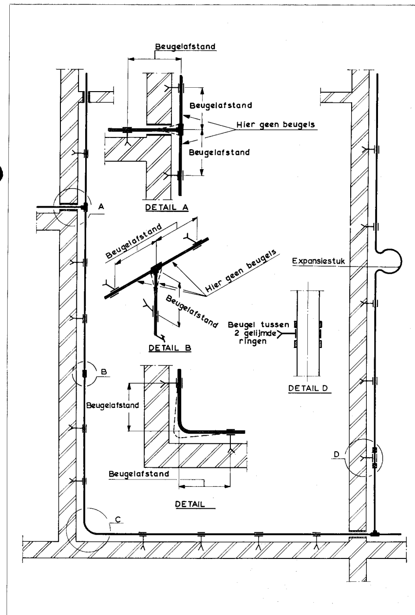
Afb. 13 - De aanleg van horizontale leidingen.
