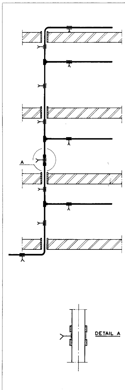
Afb. 14 - De aanleg van verticale leidingen.
