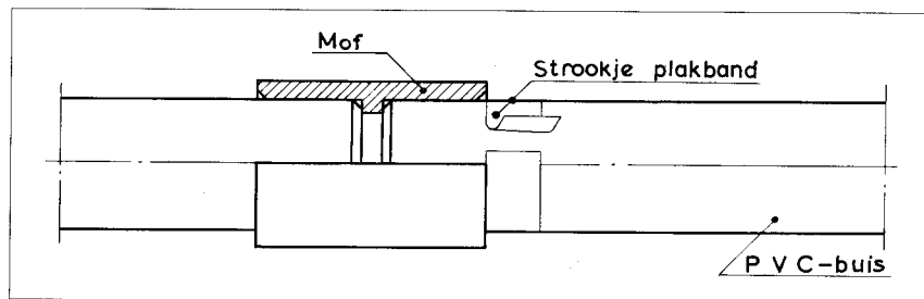
Afb. 3 - Werkwijze ter voorkoming van lijmlekken.
