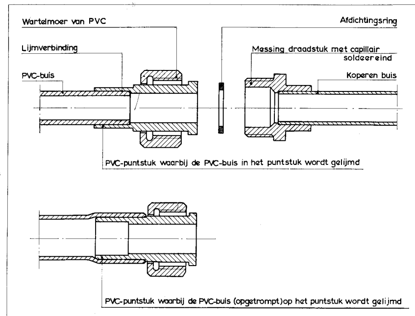
Afb. 6 - Verbindingsmethode voor de aansluiting van een PVC-buis met een puntstuk type 2 op een koperen buis.
