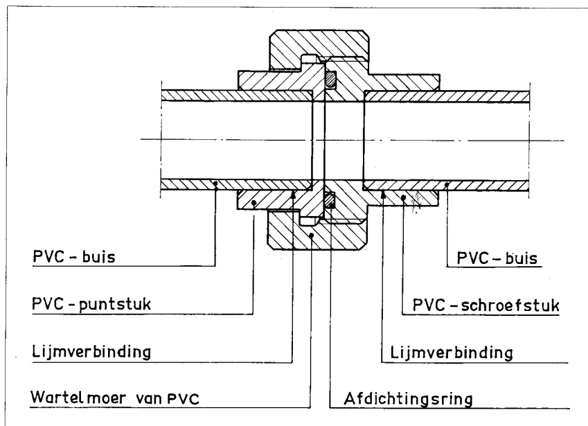
Afb. 5 - 3-delige koppeling voor een losneembare verbinding tussen twee PVC-buizen.
