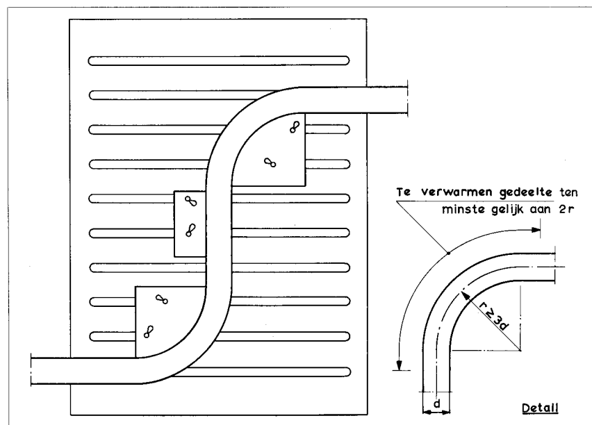
Afb. 2 - Verstelbare mal te gebruiken bij het buigen van PVC-buizen.
