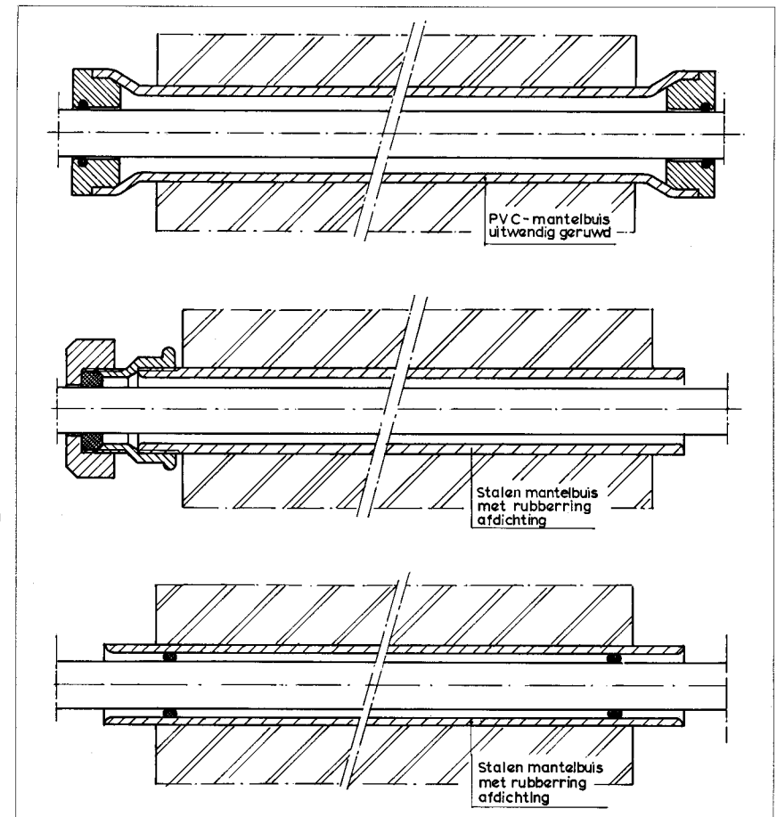
Afb. 15 - Waterdichte muurdoorvoeringen.
