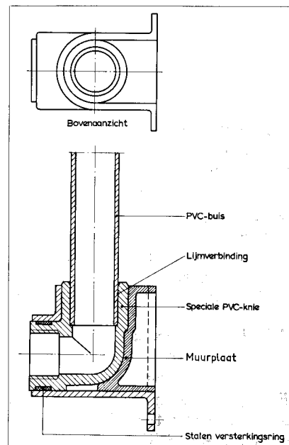
Afb. 11 - De aansluiting van een PVC-buis op een speciale muurplaat.
