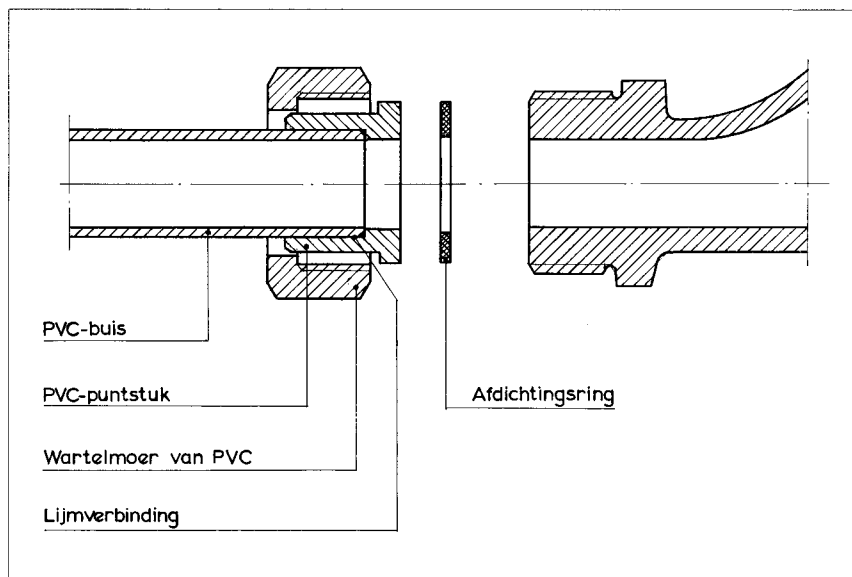
Afb. 8 - Verbindingsmethode voor de aansluiting van een PVC-buis met een puntstuk type 1 op een toestel met een aansluitende met buitendraad.
