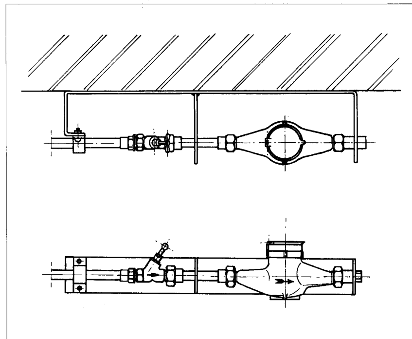
Afb. 12 - Beugel voor de ondersteuning van de watermeter en de stopkraan.
