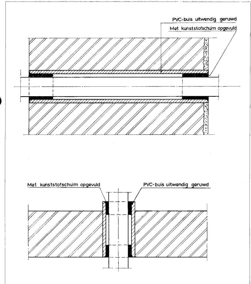
Afb. 16 - (boven) Niet waterdichte muurdoorvoering; (onder) niet waterdichte vloerdoorvoering.
