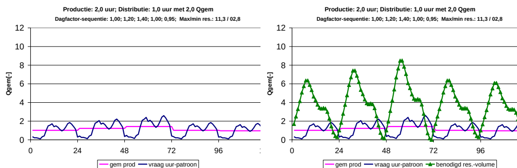
Figuur 1 Links het vraagpatroon over vijf dagen; grafiek rechts geeft het reservoirvolume behorende bij een dekking van het vraagpatroon met de gemiddelde dagproductie.
