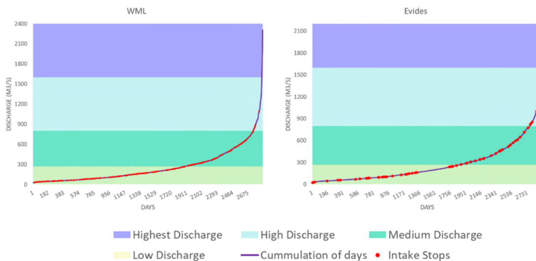
Figuur 3-3 Aantal dagen met innamestop uitgezet tegen de afvoer (data 2010-2017) van de Maas.(Duque et al, 2018).
